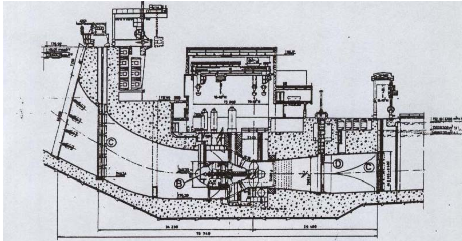
Uzdužni presjek strojárnice, A – naslage šljunka, B – cijevni agregat, C – gredne zapornice, D – brzi reg
