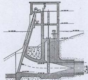
Slika 14.15. Zahvatna građevina HE Rijeka
